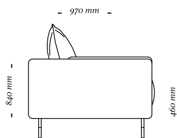
4 Lugares c/ 2 br 3140x970x840mm
