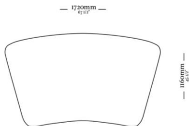
Módulo assento banquetta 101° 1720 x 1160 x 440
